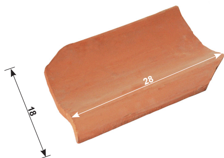
oude holle pan
